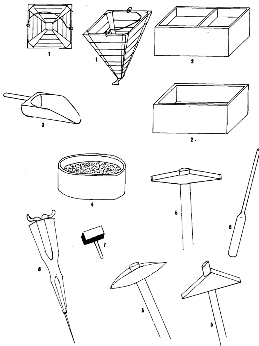
LAM. VII: Piezas accesorias del utillaje del molino
