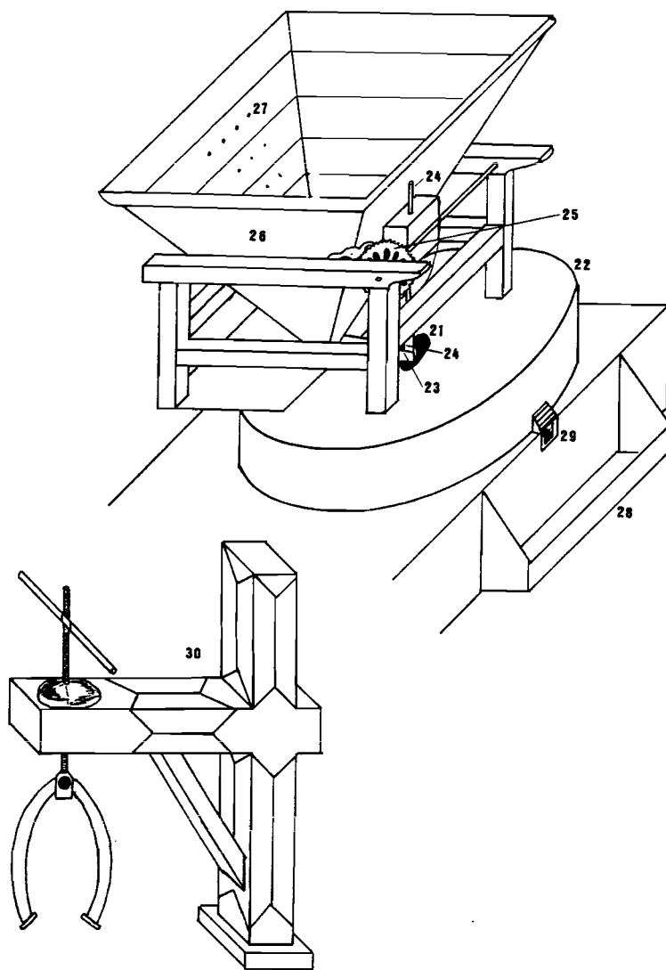
LAM. VI: Maquinaria. Tremoria, banzal y cabria
